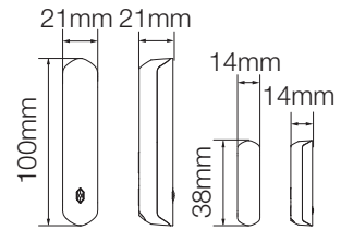
Dimensioni
