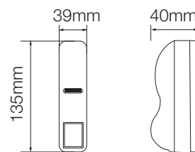
Dimensioni
