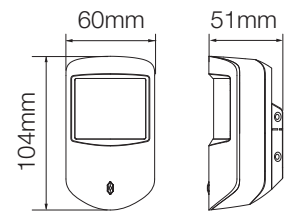
Dimensioni
