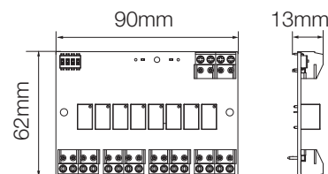
Dimensioni
