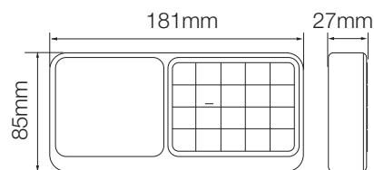
Dimensioni
