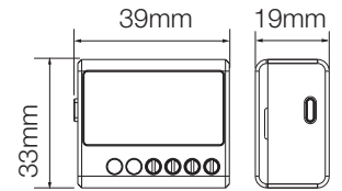
Dimensioni
